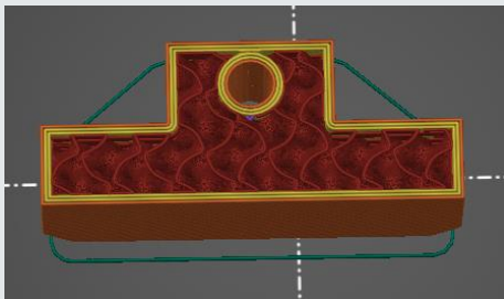
Infill 15%
